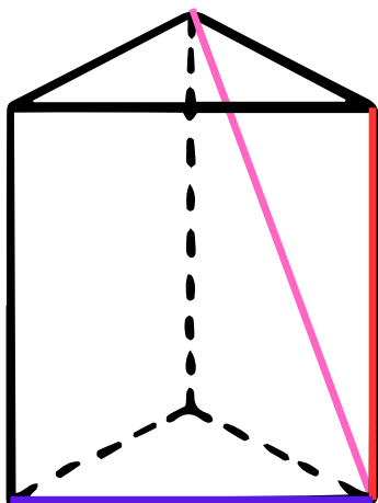
Graniastostłup trójkątny
